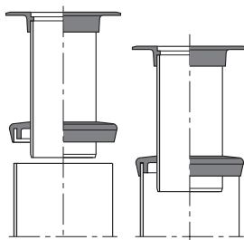
Montáž teleskopického nástavce na šachtové prodloužení.
