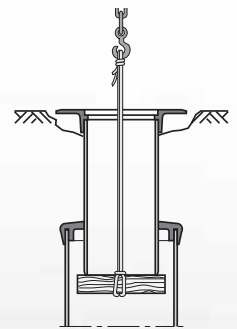
Opětovné vyzvednutí poklopů z povrchové vrstvy.
