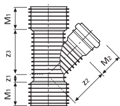
ODBOČKA UB/KG
