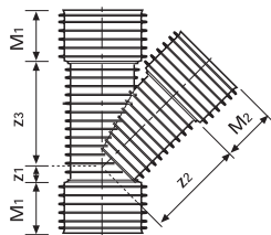
ODBOČKA UB/UB
