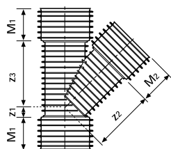
ODBOČKA UB/UB
